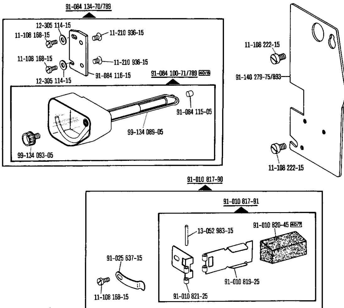
Teil zur Fadenbremse Thread retainer components Pièces du frein de fil Piezas del frenahilos
